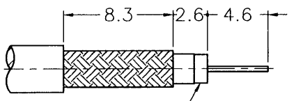
REMOVE FOIL 1mm MIN. (去除箔襯1mm以上)
